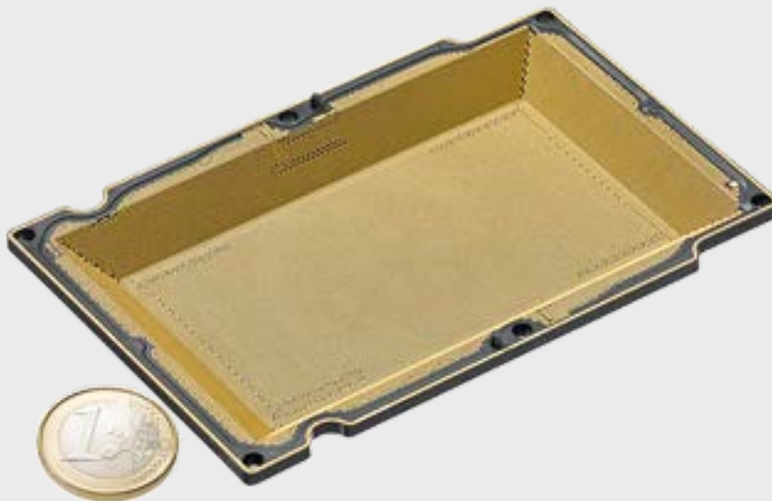
Abbildung 1: Sicherheitskappe für elektronische Zahlsysteme
