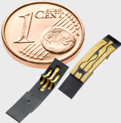
Abbildung 1: Hinter-Ohr-Hörgerät (HdO) (links) und MID-Mikrofonträger (MIC-Modul™) (rechts)
